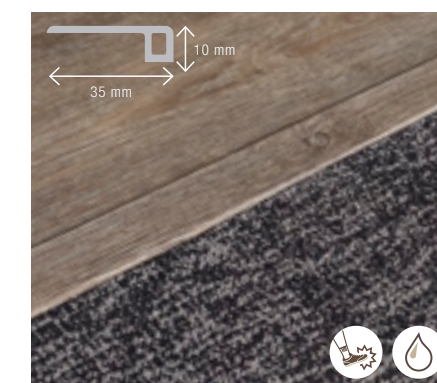
Baby Threshold / Profilé de bordure / Endprofil Eindprofil / Perfil de terminación / Profilo terminale L=240cm / 70BT3 9605 X
