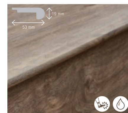
Stairnose Flush / Nez de marche / Treppenkante Trapneus / Mamperlán / Profilo toro per gradino L=240cm / 70SN3 9605 X
